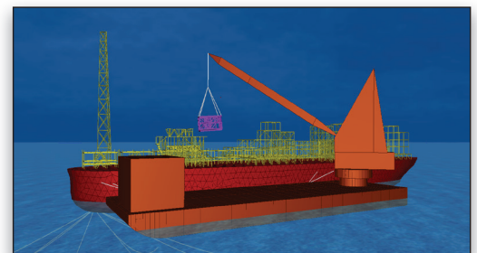
Simulação de Lançamento com Multi Corpos
